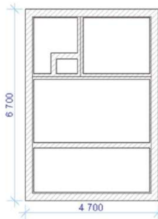
План фундамента
